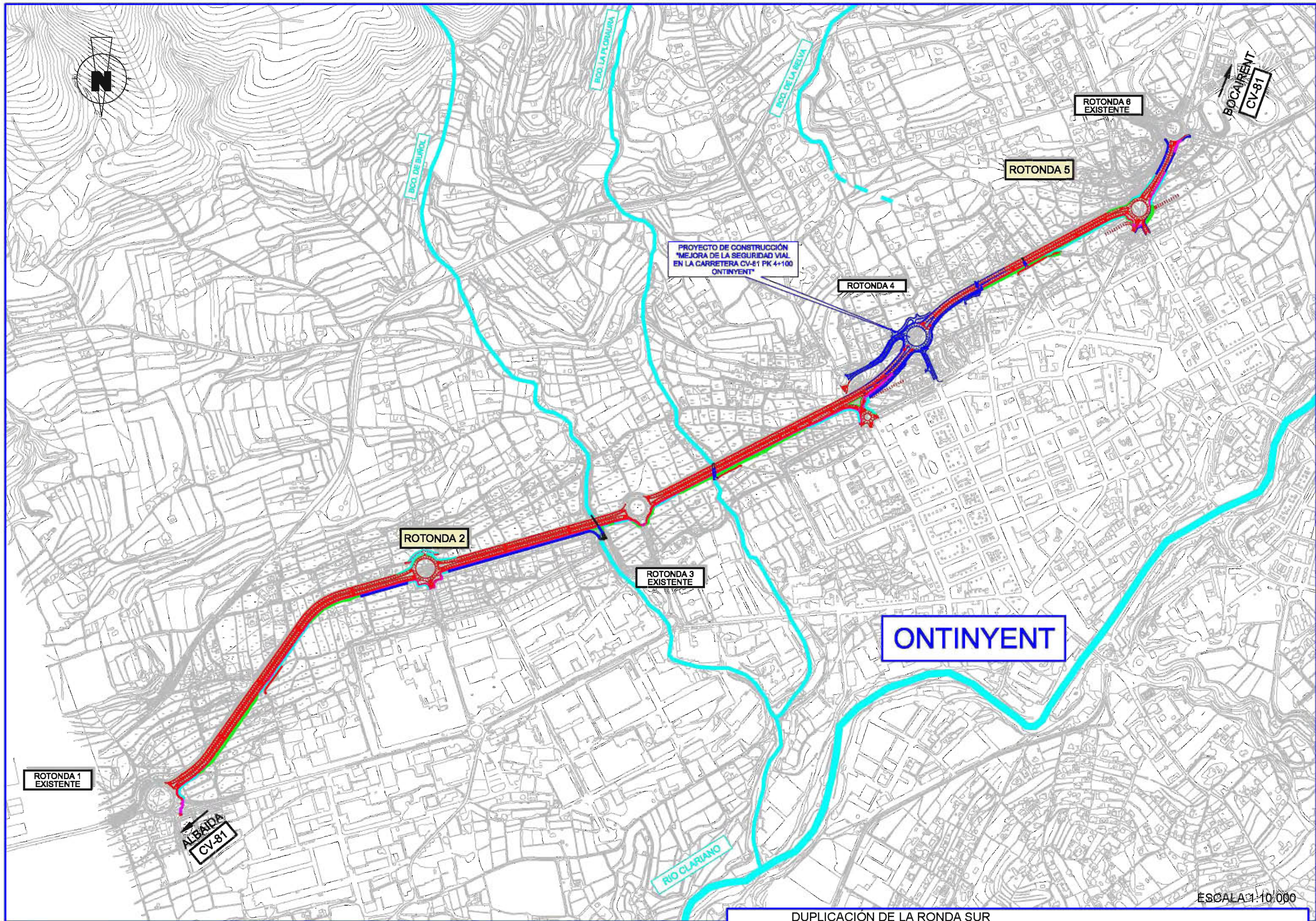
2. PLANTA GENERAL
